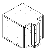
DA-1/N Elemento DA+DO nobilitato DA+DO element in faced panel L. 38,5 x P. 40 x H. 40 cm
