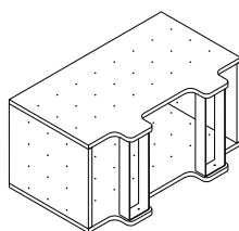
DA-2/N Elemento DA+DO nobilitato DA+DO element in faced panel L. 76,5 x P. 40 x H. 40 cm
